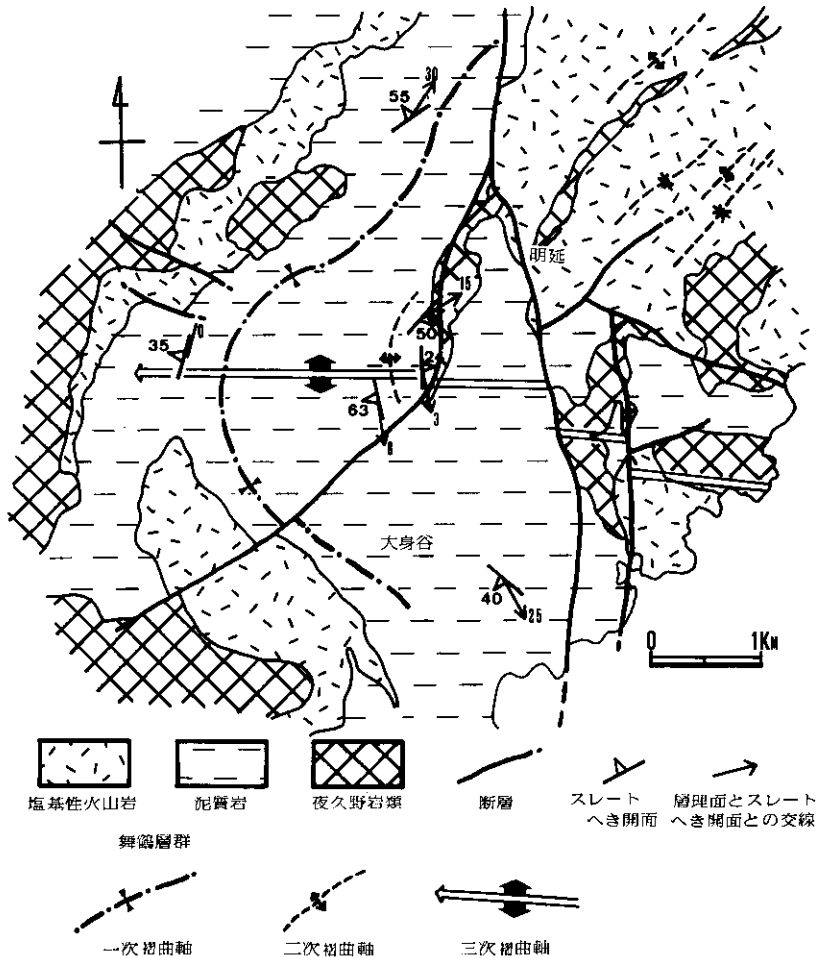
第4図 明延地域の舞鶴層群の構造図（金属探鉱事業団，1973および SATO & AKIYAMA，1980による）
