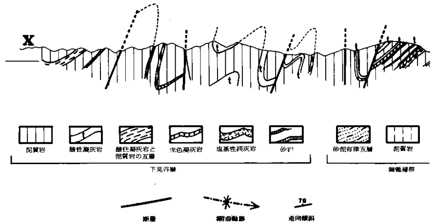
第2図 志高地域の地質断面図
