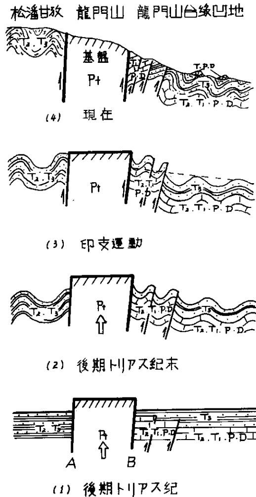
図16 龍門山飛来峰の形成模式図
