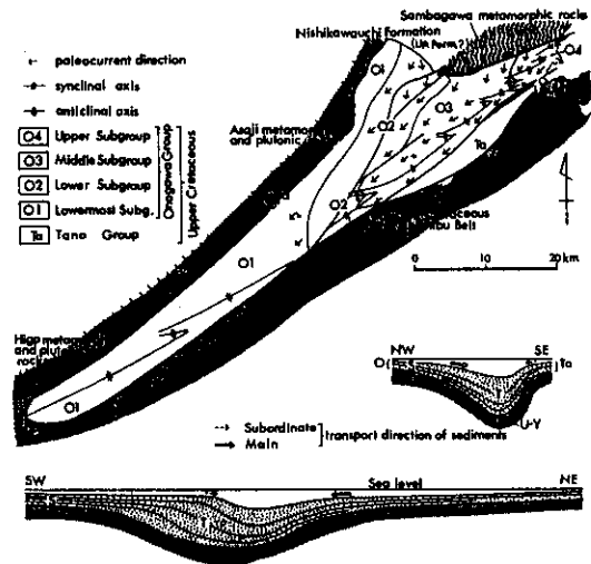
第11図 大野川層群の古流系と堆積モデル(寺岡, 1977). Ta: 田野層群, O: 大野川層群, U-Y: 白杵—八代構造線, S: 陸棚相, T: 主にタービダイト相。
