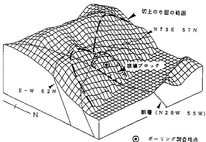
第8図 崩壊のり面の鳥瞰図(最大キープブロックによる斜面の崩壊例)
