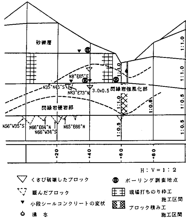
第9図 のり面の状況 西垣ほか(1989)
