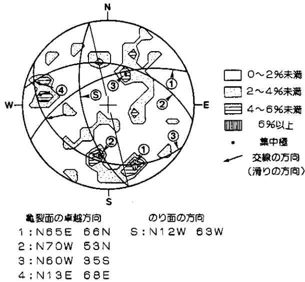
第10図 亀裂面の方向の密度分布 西垣ほか(1989)
