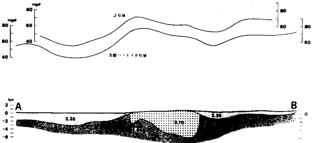
図4 断面図
