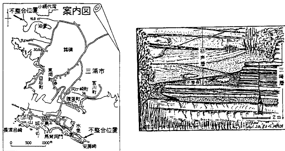
図-1 油壺における中新世三崎層と初声層との不整合
